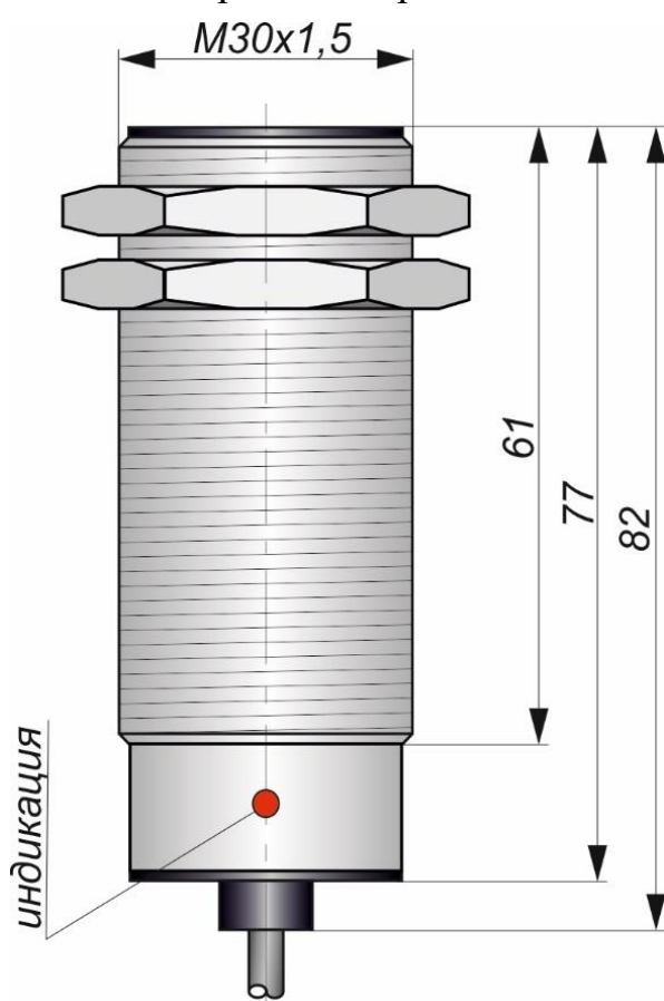
Габаритный чертеж
