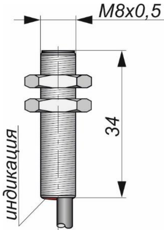
Габаритный чертеж
