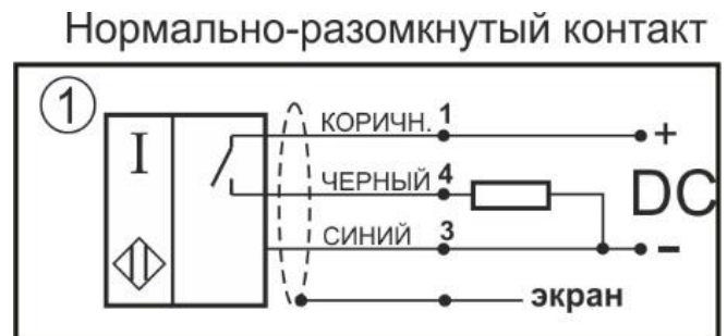
Схема соединения
