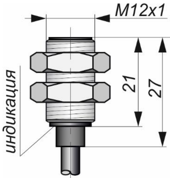
Габаритный чертеж
