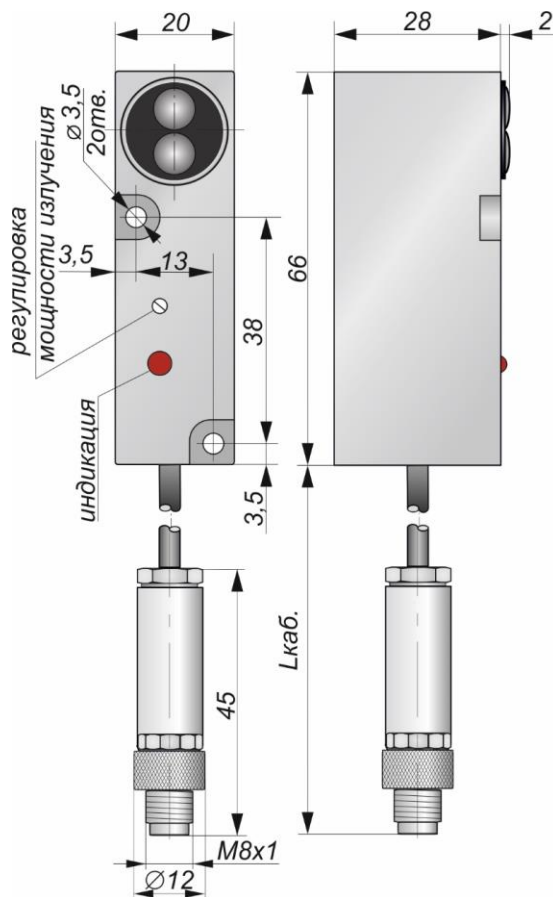
Габаритный чертеж
