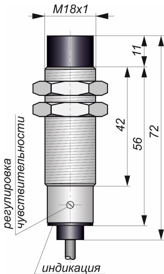
Габаритный чертеж
