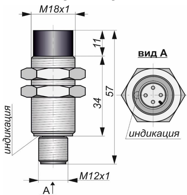
Габаритный чертеж
